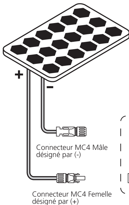
La Fig 4.1 Connexion des câbles d'extension aux câbles de sortie du panneau solaire
