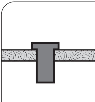
La Fig. 3.5. L'écrou-douille est inséré dans un trou pré-percé avec sa bride contre la surface extérieure. Il n'est pas nécessaire d'accéder à la surface intérieure.
