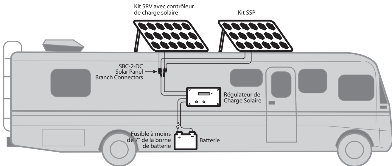
La Fig. 3.1. Bloc-Diagramme de l'installation
