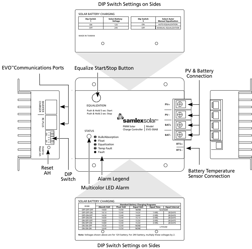
Fig. 5.1. EVO-30AB Layout
