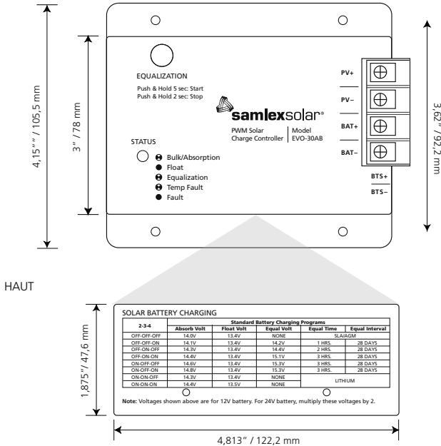
La Fig. 6.1. Dimensions de l'EVO-30AB
