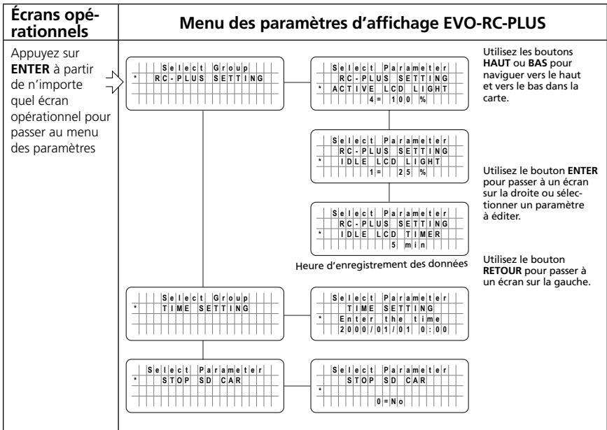
Figure 5.4 : Carte des menus EVO-RC-PLUS et EVO-30AB
