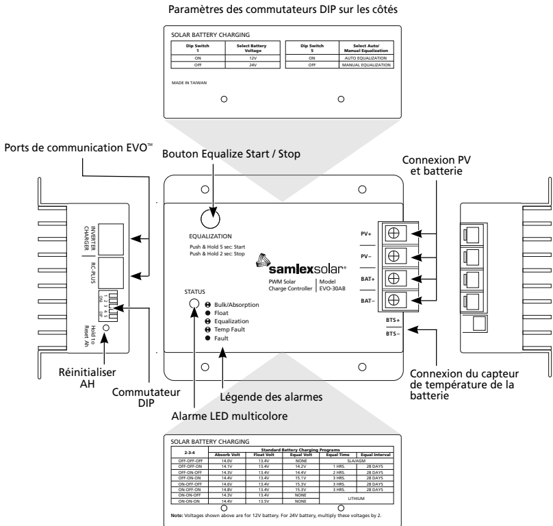
Fig. 5.1. Disposition EVO-30AB
